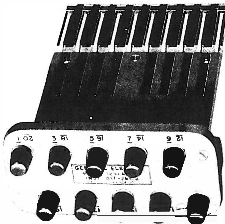
Fig. 2 XLA13A Test Plug
