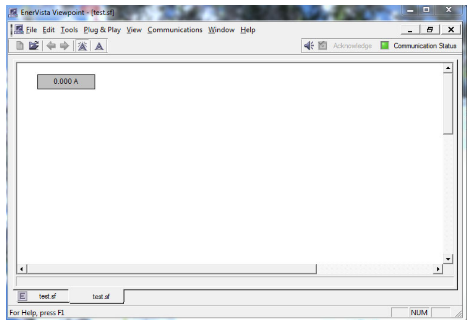
Figure 119: Parameter display
