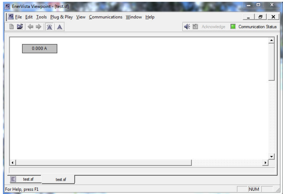
Figure 104: Parameter display
