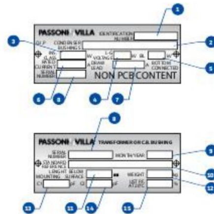
Fig. 12b: Nameplate
