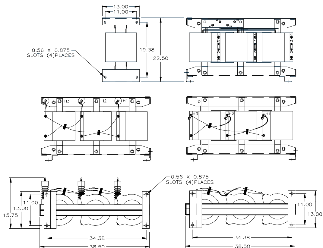
Dimensions for 95kV BIL units
