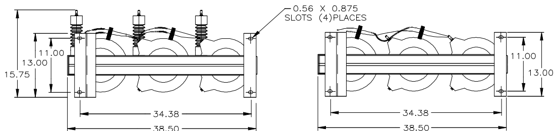
Dimensions for 95kV BIL units
