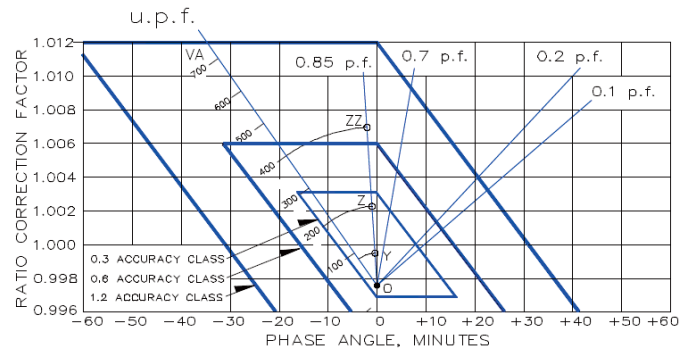
CIRCLE DIAGRAM
