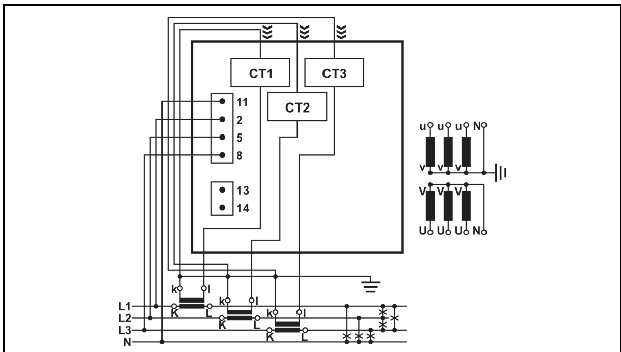
FIGURE 16-6 : SCHEMA DE CABLAGE EXTERNE : CONNEXION TRIPHASEE, 4 FILS AVEC CHARGE DESEQUILIBREE (4U)
