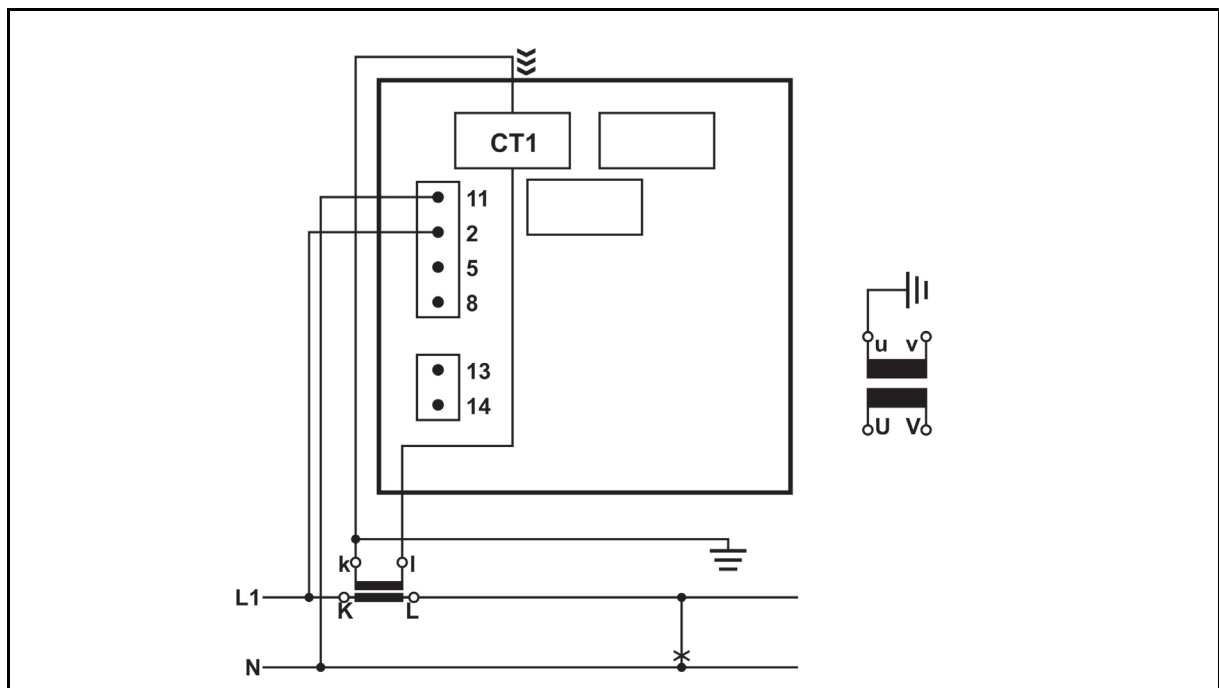
FIGURE 16-2 : SCHEMA DE CÂBLAGE EXTERNE : CONNEXION MONOPHASEE (1B)
