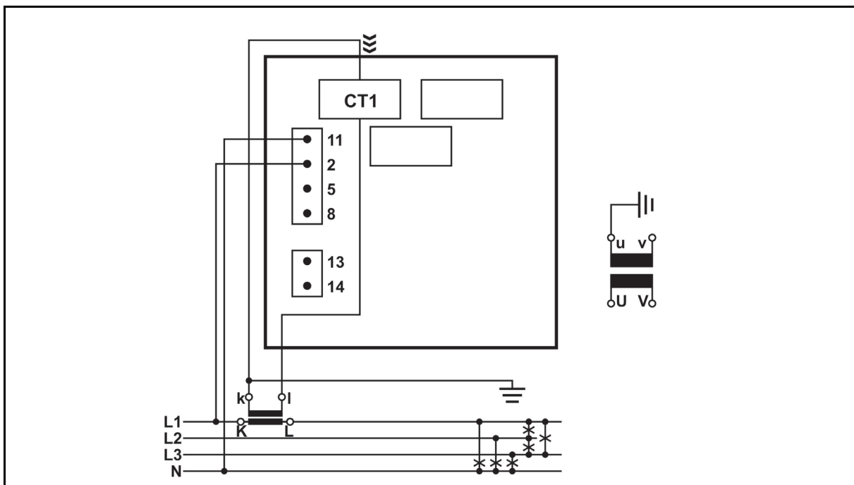
FIGURE 16-4 : SCHEMA DE CABLAGE EXTERNE : CONNEXION TRIPHASEE, 4 FILS AVEC CHARGE EQUILIBREE (4B)
