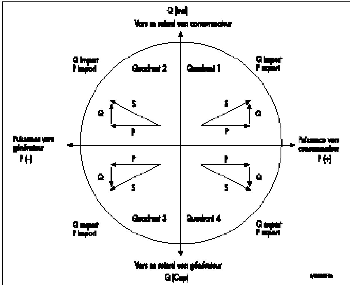
FIGURE 8-1 : FLUX D'ÉNERGIE
