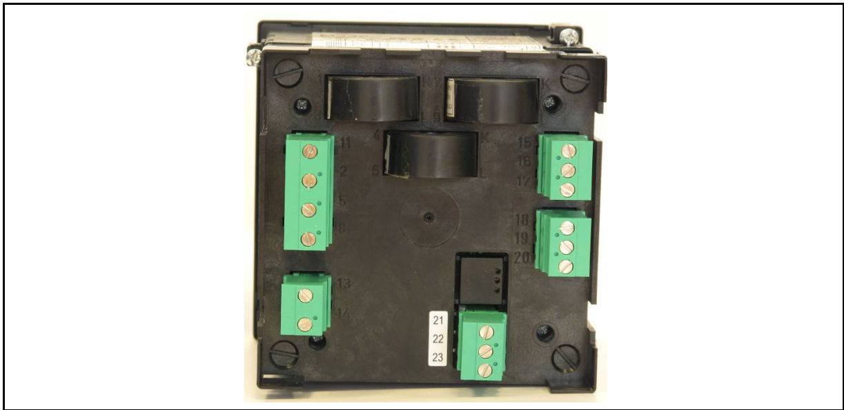
FIGURE 10-1 : VUE ARRIERE DU BOITIER M2X2
