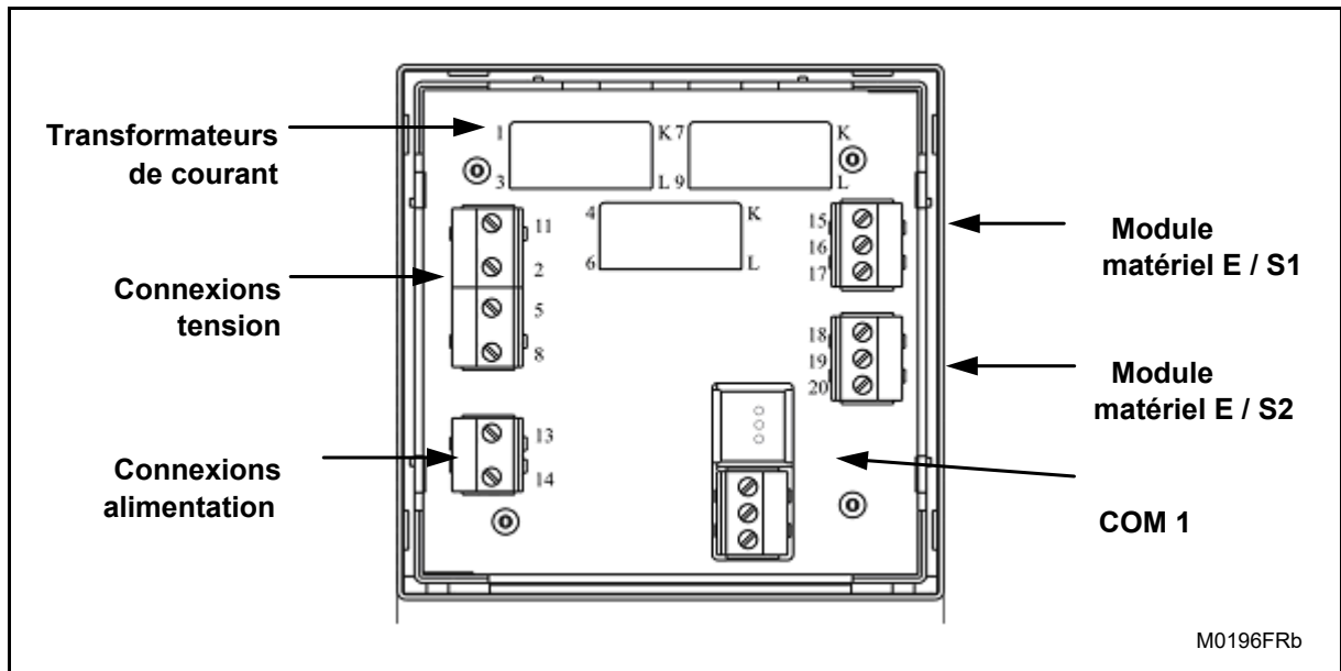
FIGURE 16-1 : CONNEXIONS
