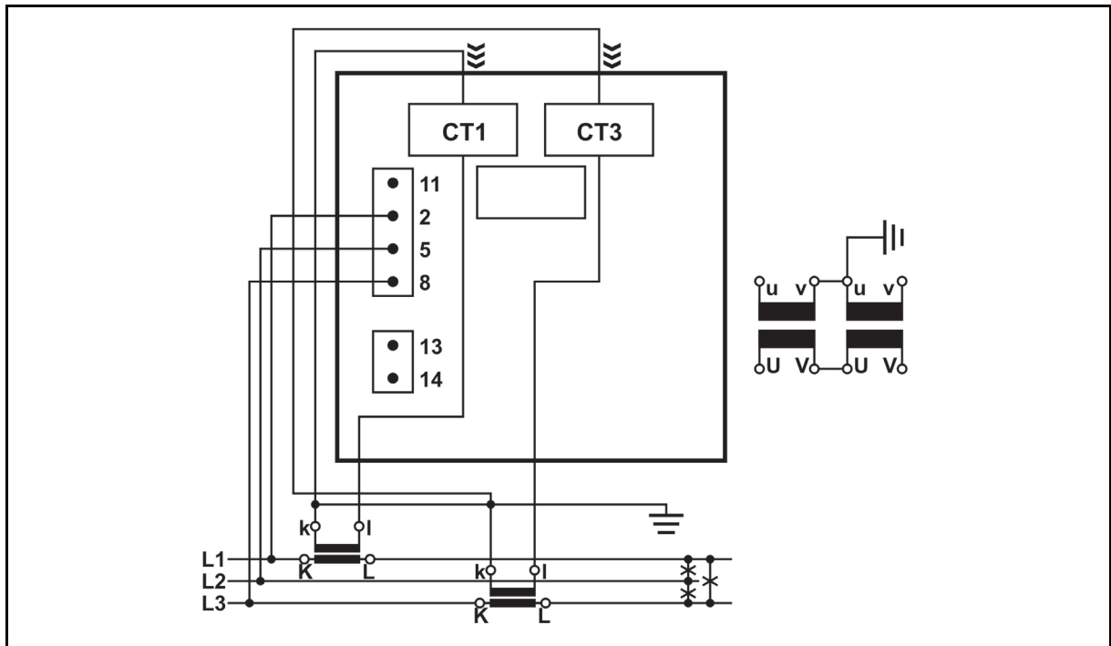
FIGURE 16-5 : SCHEMA DE CABLAGE EXTERNE : CONNEXION TRIPHASEE, 3 FILS AVEC CHARGE DESEQUILIBREE (3U)
