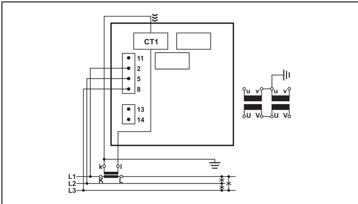
FIGURE 16-3 : SCHEMA DE CABLAGE EXTERNE : CONNEXION TRIPHASEE, 3 FILS AVEC CHARGE EQUILIBREE (3B)
