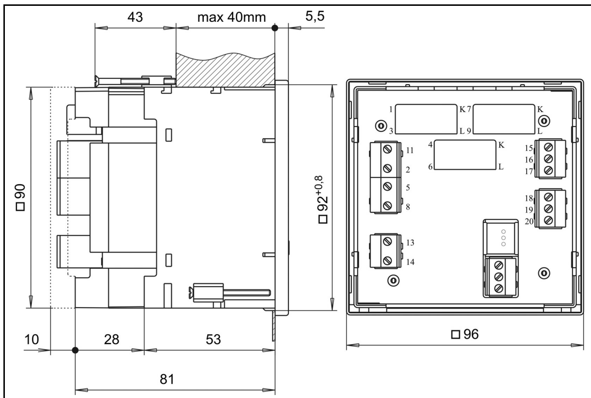
FIGURE 16-8 : DIMENSIONS DU BOITIER
